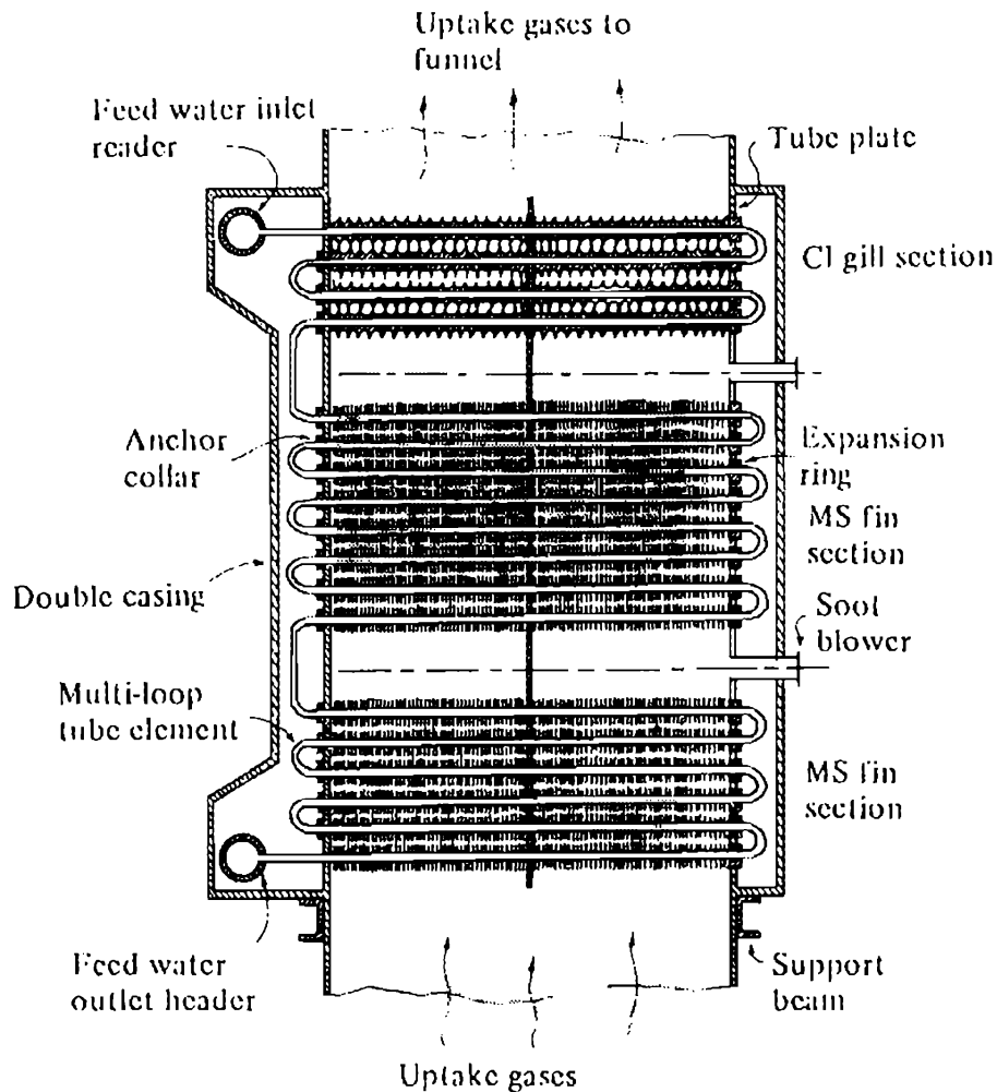
Fig. 52 Economiser
