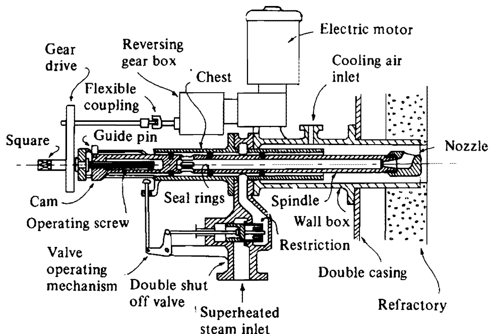
Fig. 78 Soot blower
